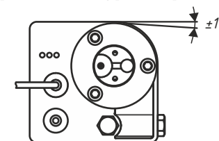
Рис.2. Ориентация датчика для контроля нижнего уровня
