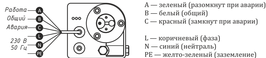
Рис.3. Электрические соединения
