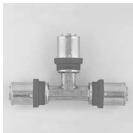
Номер по каталогу и название 25130 – тройник НПр
