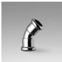
Номер по каталогу и название 16041 – отвод 45°, ВПр-ВПр
