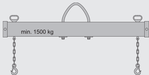
Рис. 1 Подъем компрессора
